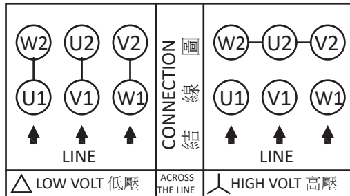
6 條結線 6 Lead
