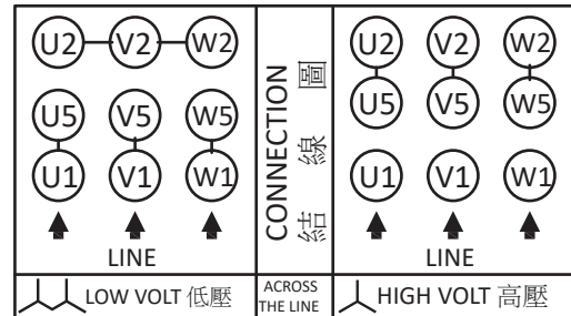
9 條結線 9 Lead
