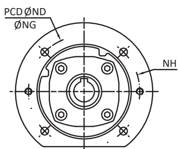
IEC-B5
